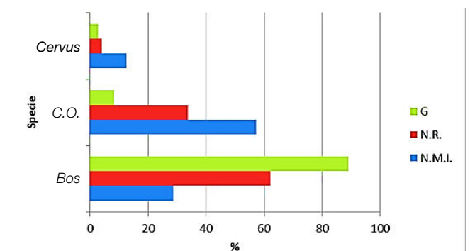
Fig. 4 - NISP for each species identified for period B (Early-Middle Bronze Age). / Rappresentazione del lotto faunistico relativo al periodo B (Età del Bronzo antica-media).
